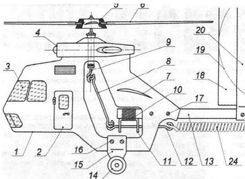
Рис. 2. Кабина пилота.
