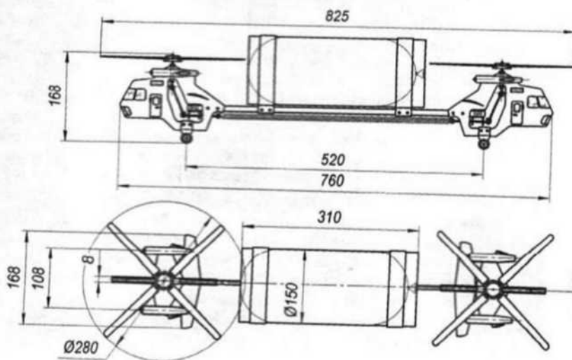
Рис. 1. Общий вид модели.
