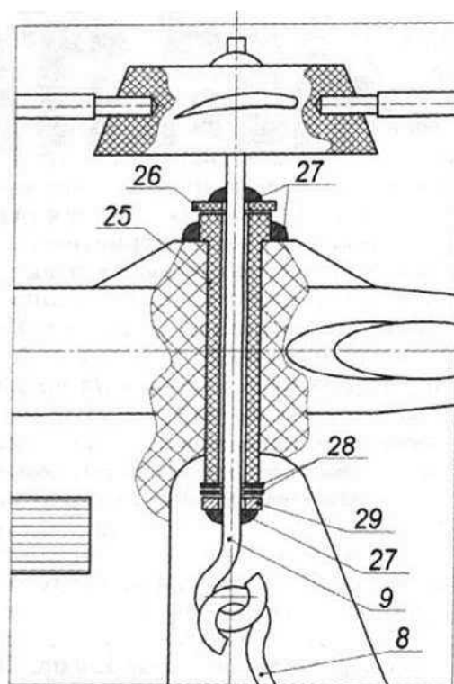
Рис. 5. Схема установки ротора.
